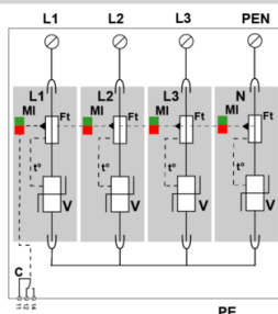
V: высокоэнергетический варистор Ft: тепловой предохранитель C: Контакт дистанционного сигнала t °: Система термического отключения MI: индикатор отключения
